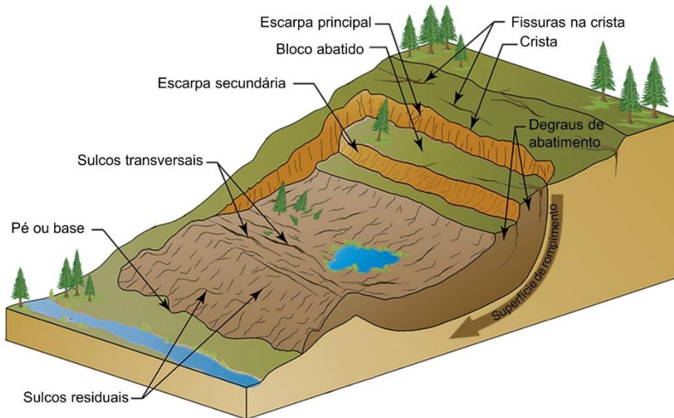
Figura 50 – Esquema dos escorregamentos circulares ou rotacionais.
