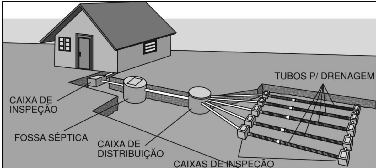
Figura 35 - Sistemas de tratamento individual- Valas de Infiltração.
