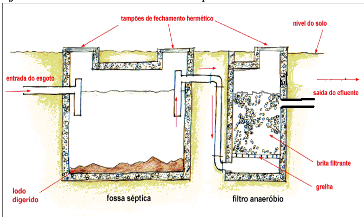
Figura 34 - Sistema individual de tratamento - Fossas Sépticas.
