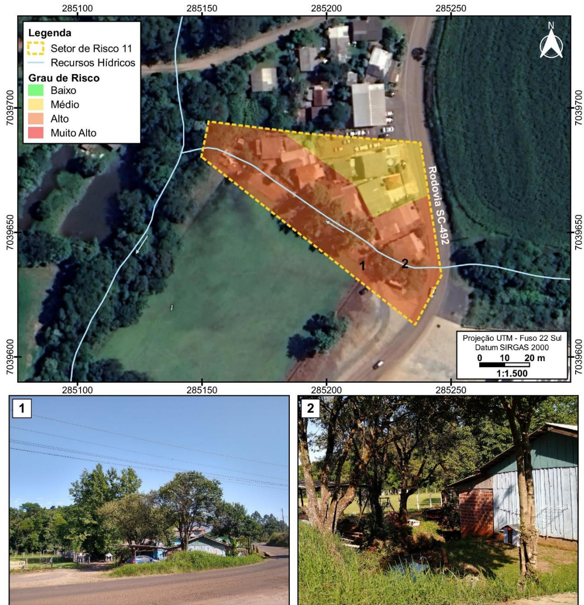
Figura 81 - Classificação de Risco do Setor 11 e fotografias da área: 1) Vista geral da ocupação no setor; 2) Proximidade das moradias ao curso d'água, colocando as mesmas em risco em épocas de chuvas intensas, devido a possibilidade de ocorrência de enxurradas.
