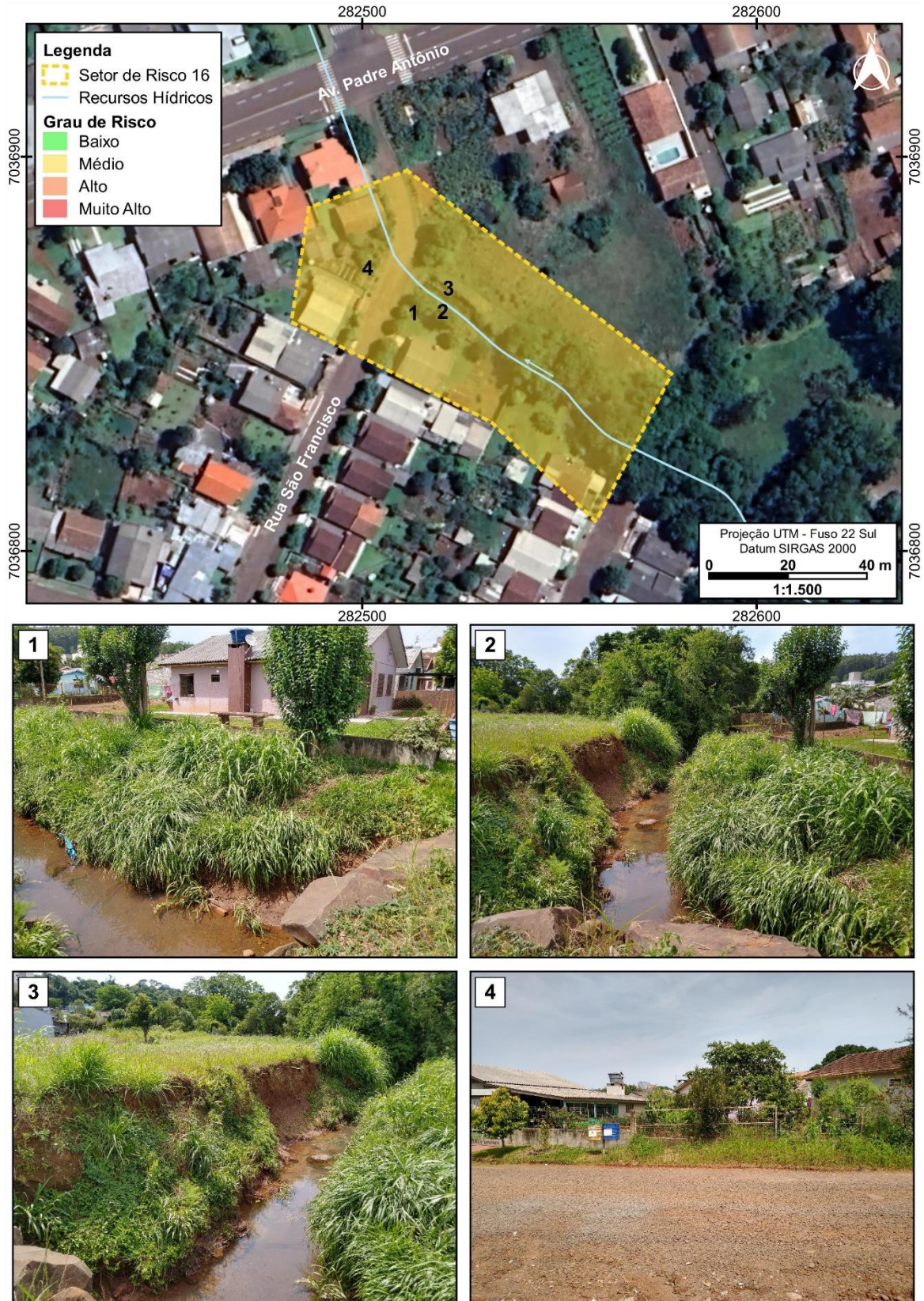
Figura 86 - Classificação de Risco do Setor 16 e fotografias da área: 1, 2 e 3) Vista geral do leito e da ocupação ao longo do trecho aberto, com ocorrência de deslizamentos na margem; 4) Vista da ocupação no trecho tubulado.
