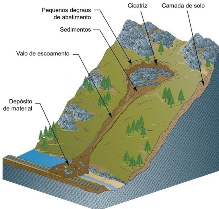
Figura 52 – Esquema do movimento de massa do tipo corrida.
