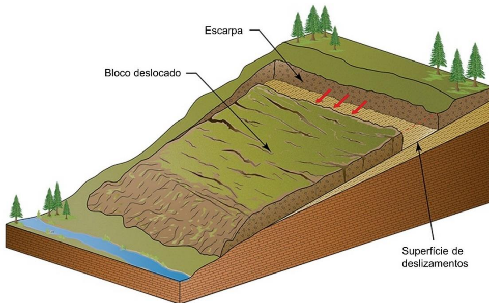
Figura 49 – Esquema dos escorregamentos planares ou translacionais.
