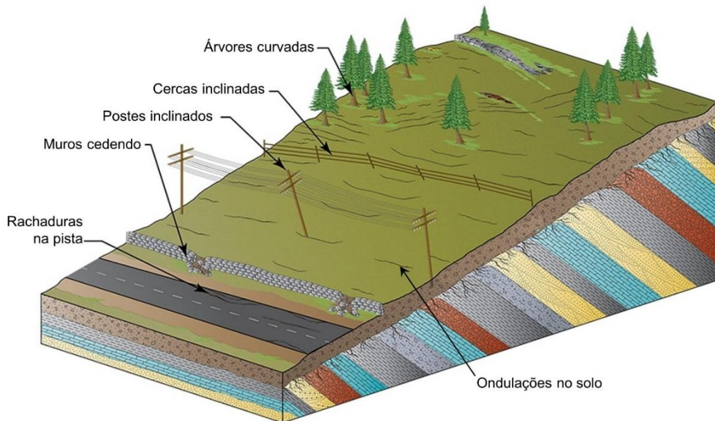
Figura 48 – Esquema do movimento de massa do tipo Rastejo.
