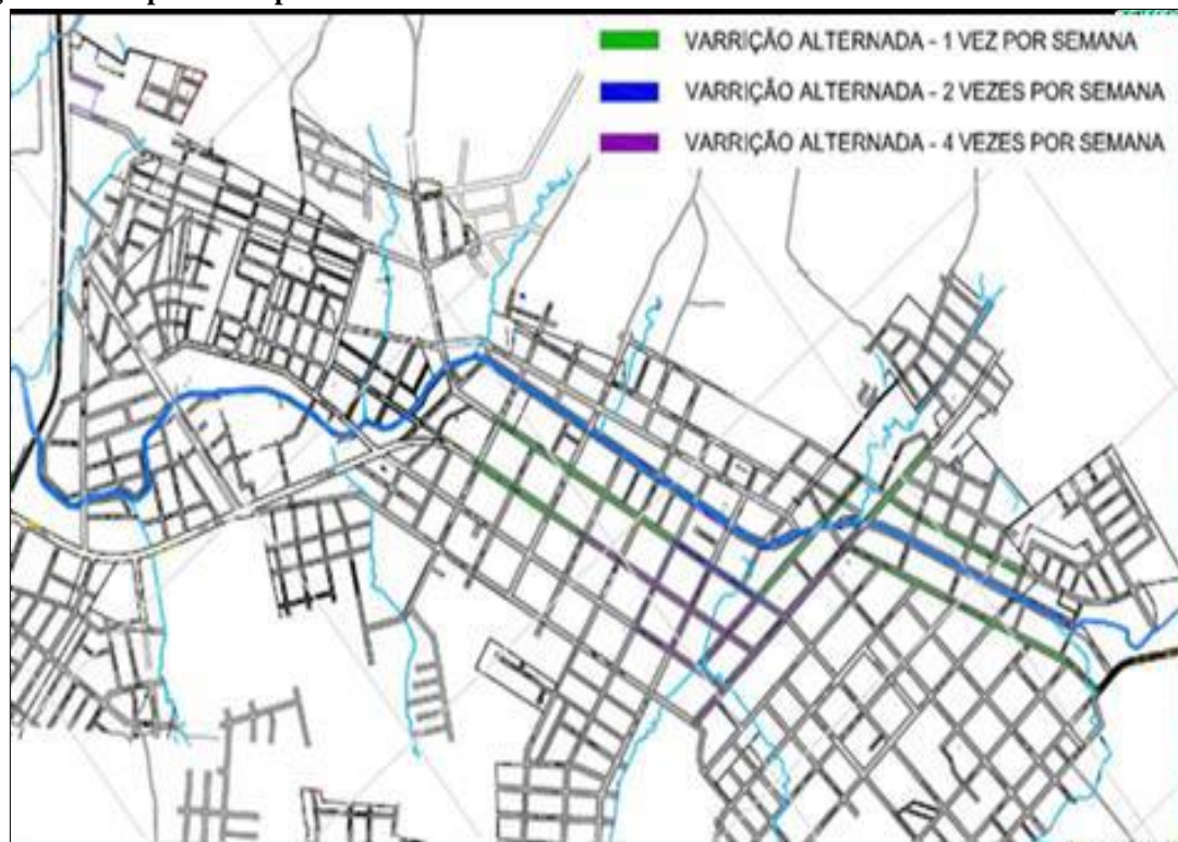
Figura 45 – Mapa da Limpeza Urbana.
