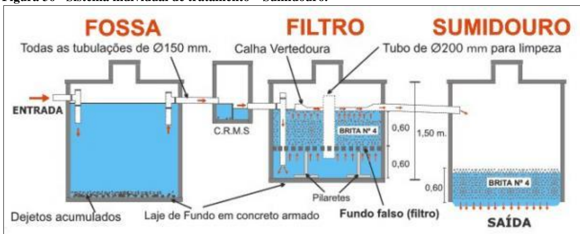
Figura 36 - Sistema individual de tratamento – Sumidouro.
