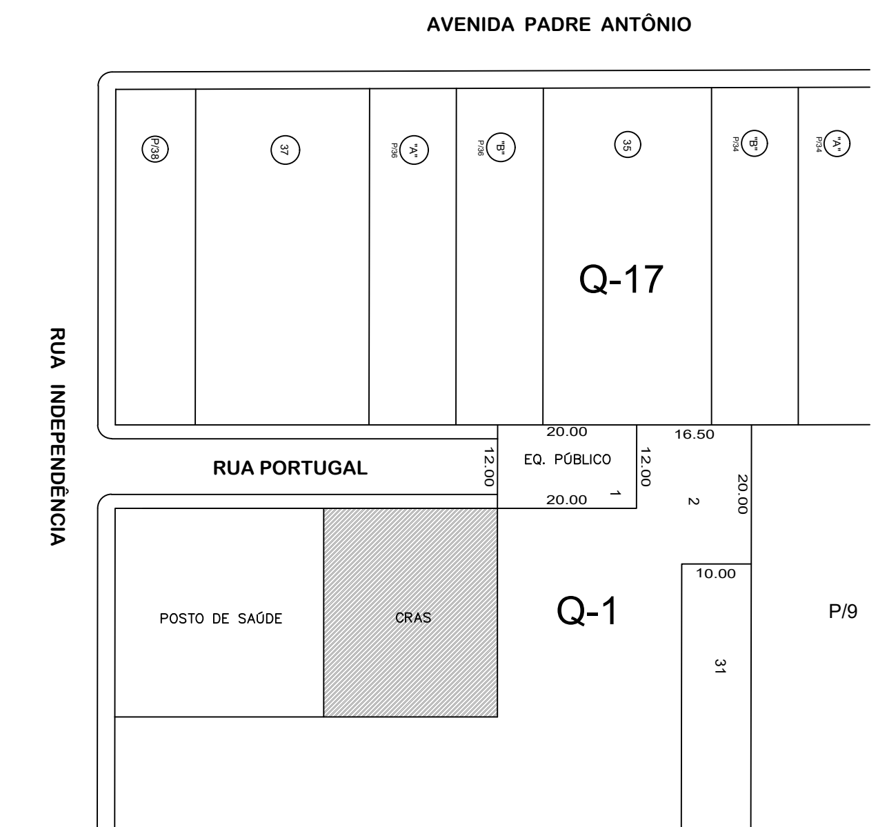
PLANTA SITUAÇÃO ESC.: 1:750
