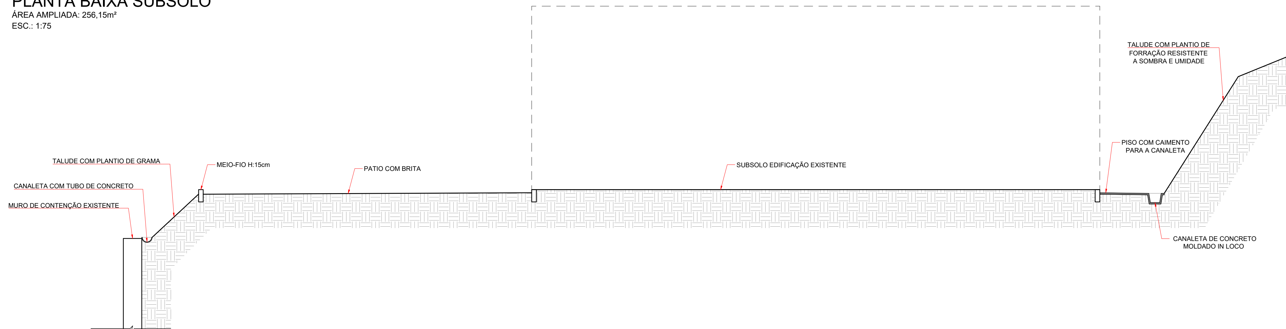
CORTE AA PERFIL PROPOSTO PARA O TERRENO ESC.: 1:75
