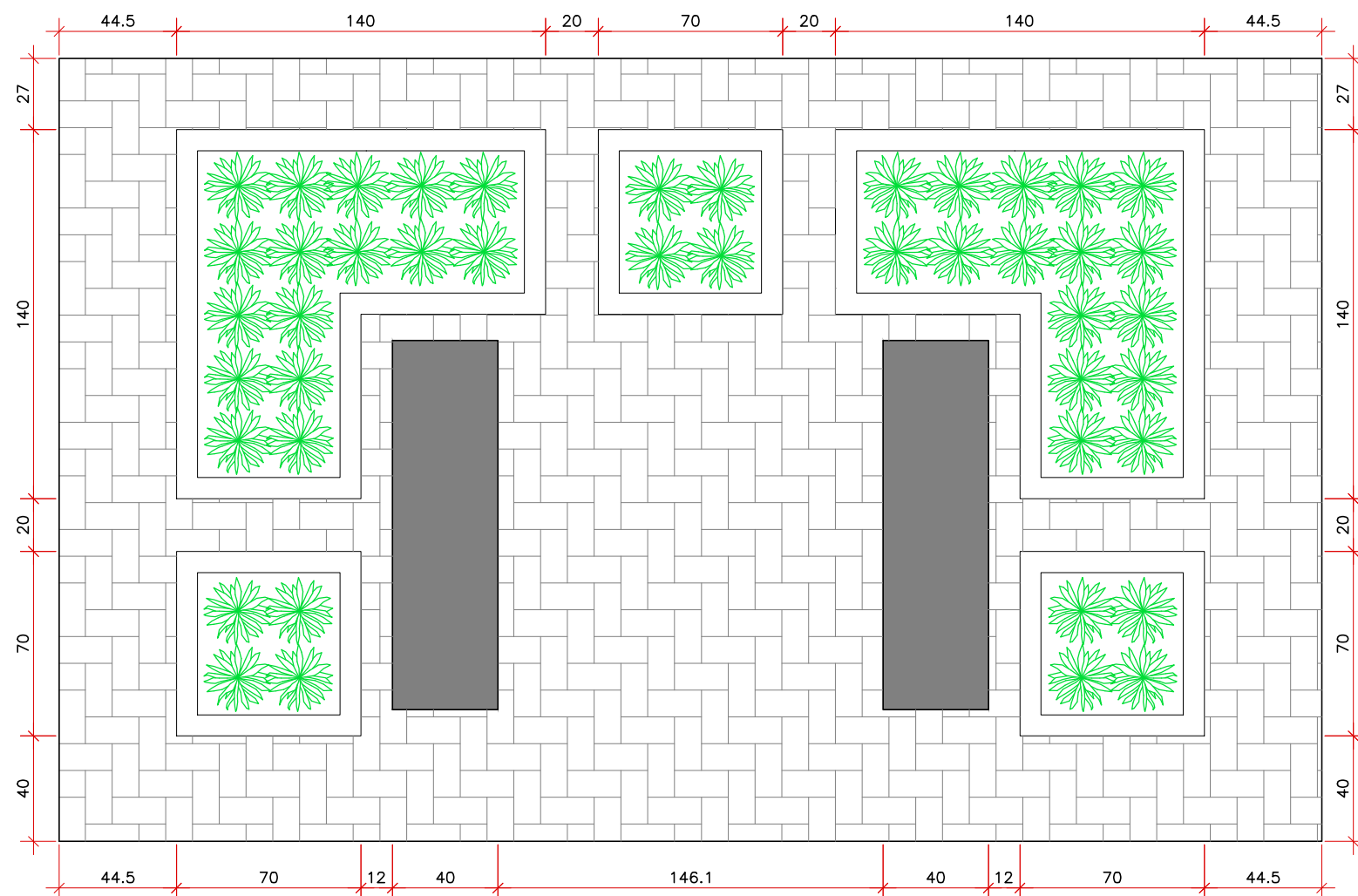
PLANTA DE LOCAÇÃO DO PARKLET Esc.:1/25
