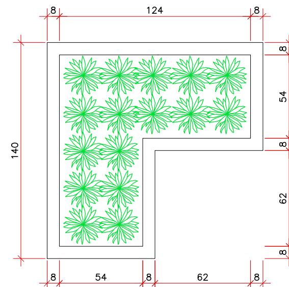
PLANTA BAIXA FLOREIRA TIPO 01 Esc.:1/25
