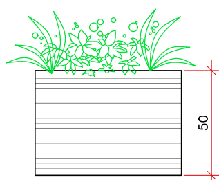
VISTA FLOREIRA TIPO 03 Esc.:1/25
