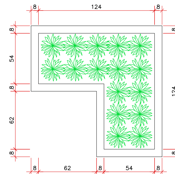
PLANTA BAIXA FLOREIRA TIPO 02 Esc.:1/25
