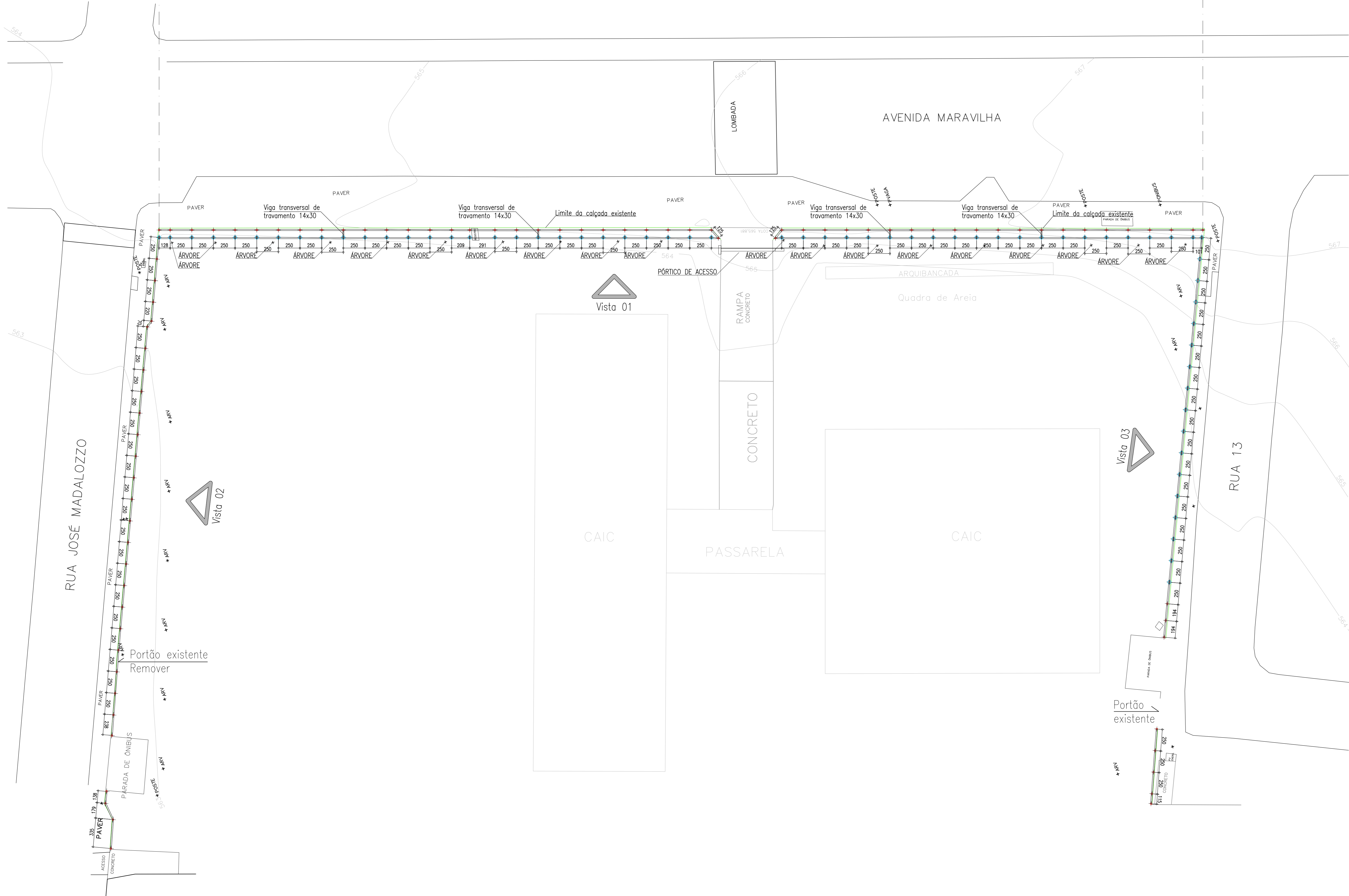
Localização: Cercamento + Pórtico Unidade de medida (cm) Escala: 1:200
