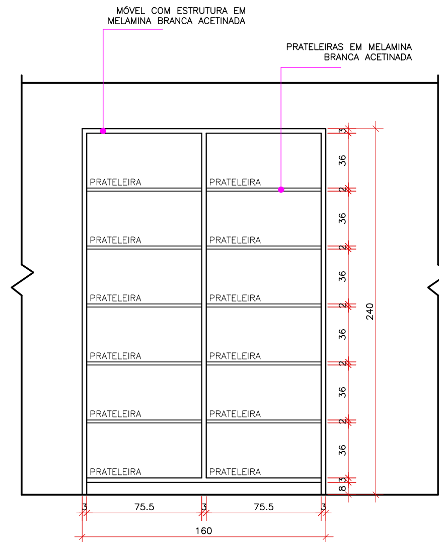
VISTA K - MÓVEL 06
