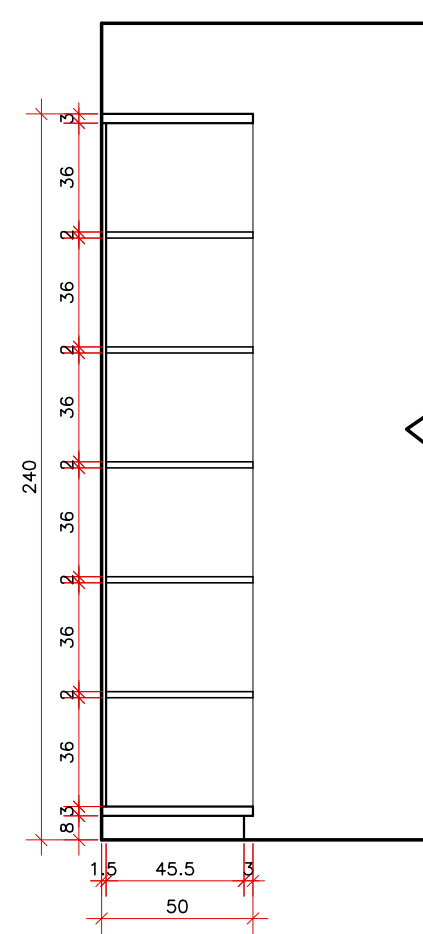
CORTE L - MÓVEL 06
