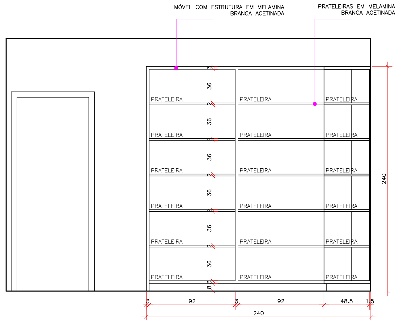
VISTA I - MÓVEL 05
