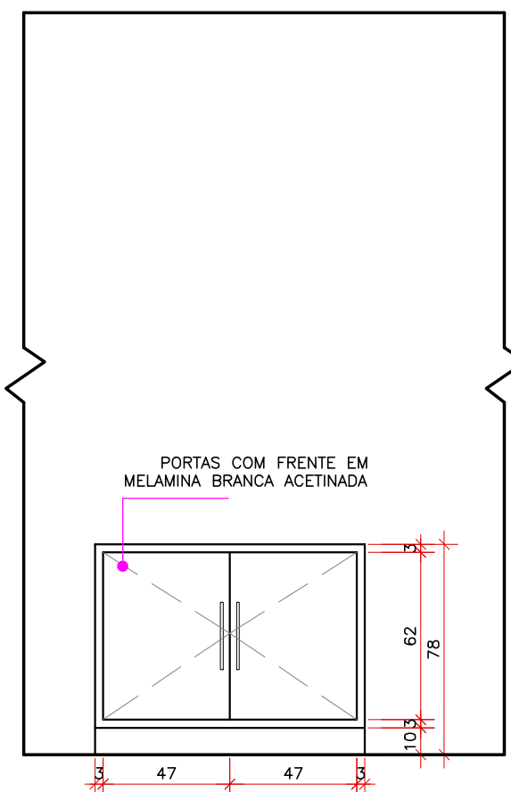
VISTA F - MÓVEL 04 Esc.:1/25
