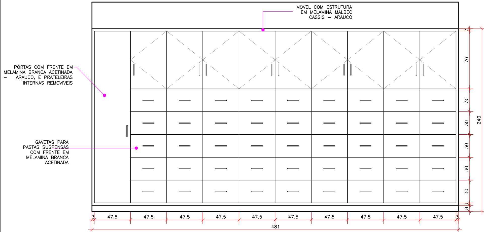
VISTA A - MÓVEL 01 Esc.:1/25
