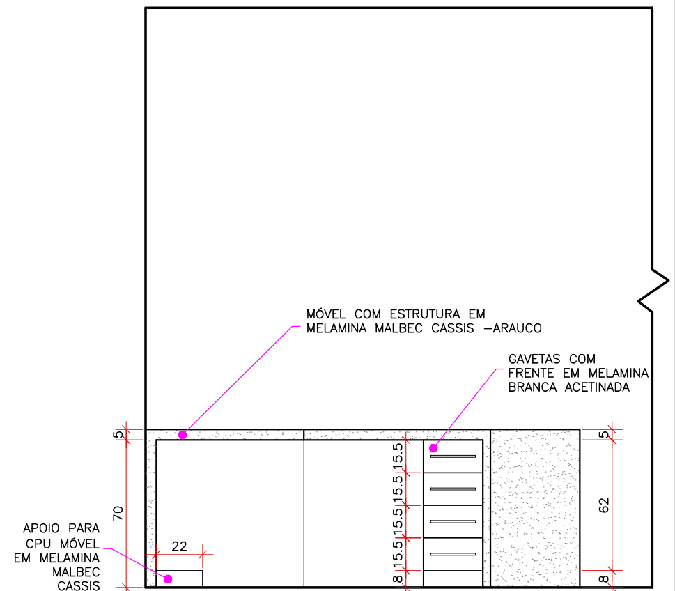
VISTA C - MÓVEL 02 Esc.:1/25
