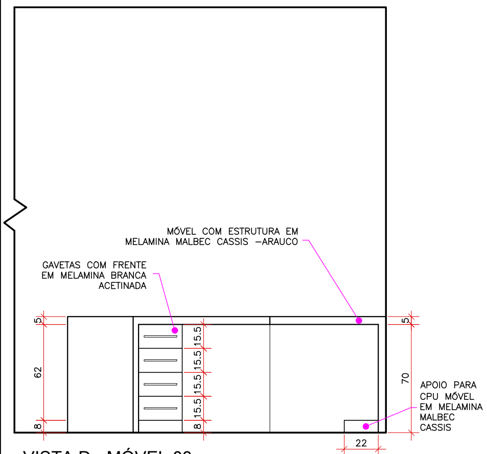
VISTA D - MÓVEL 03 Esc.:1/25
