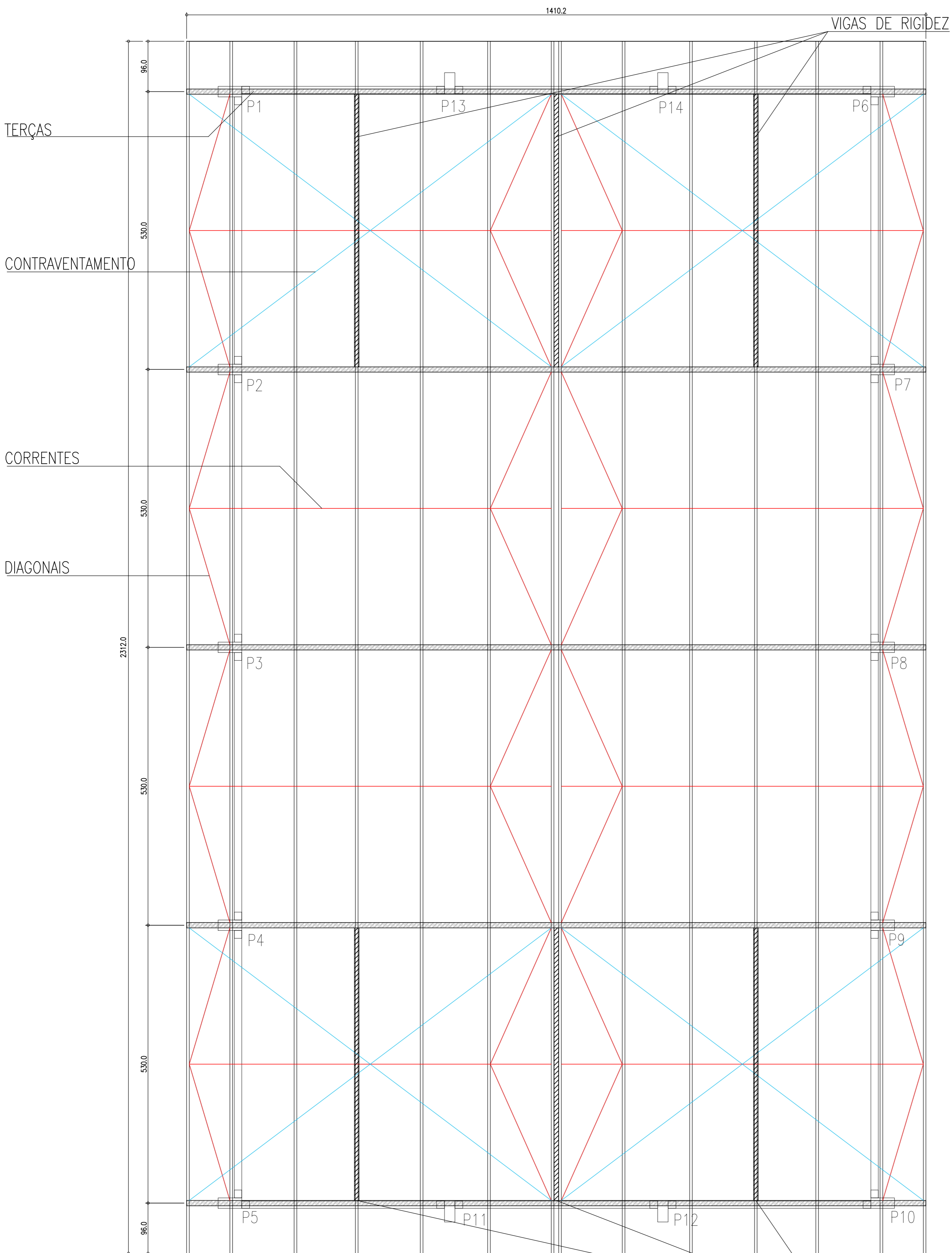
Planta baixa: Estrutura metálica de cobertura Escala: 1:50
