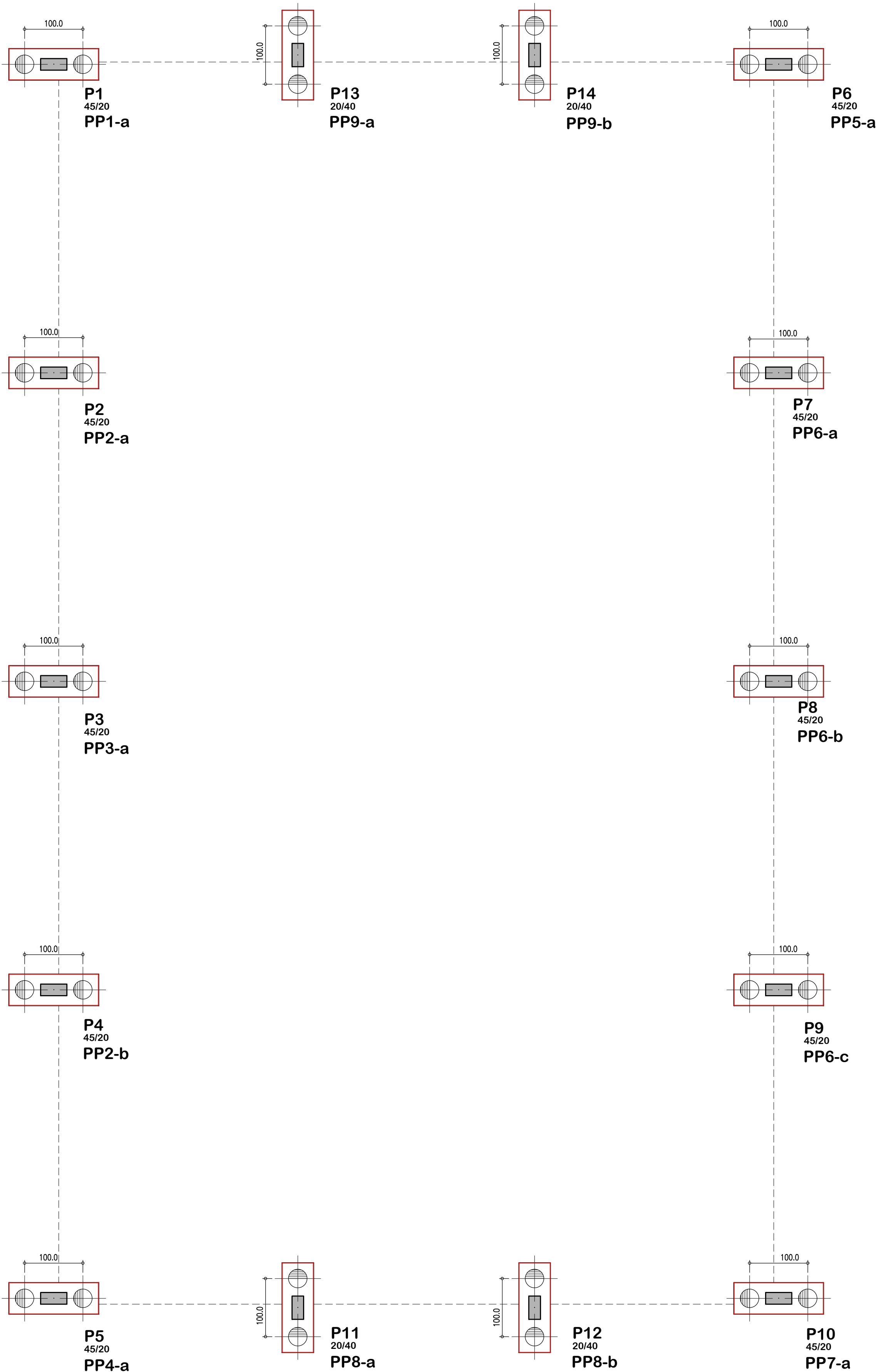
Y X Planta: Locação das estacas Escala: 1:50
