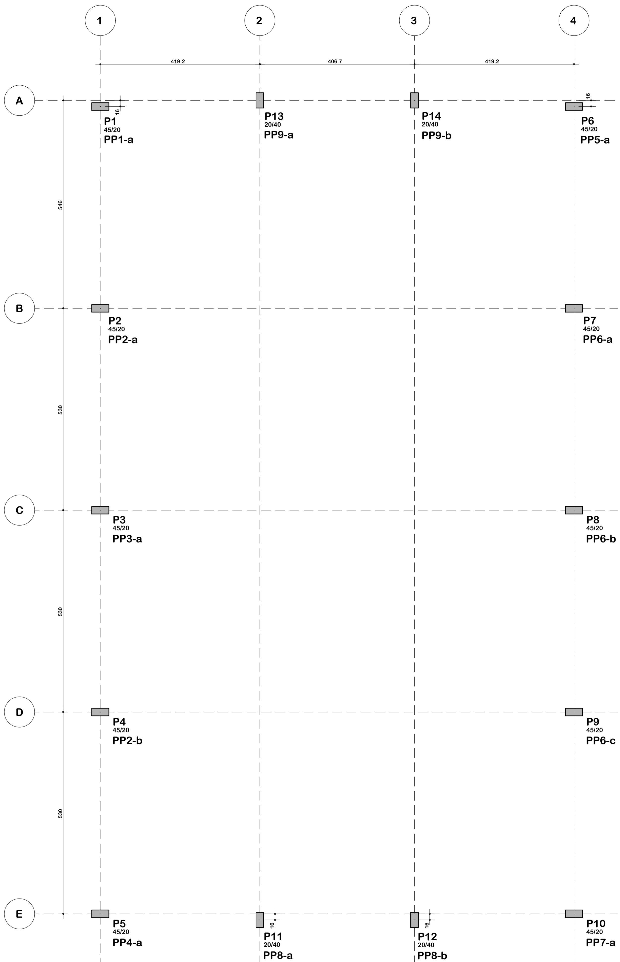
↑ Y ↓ X Planta: Locação dos pilares Escala: 1:50
