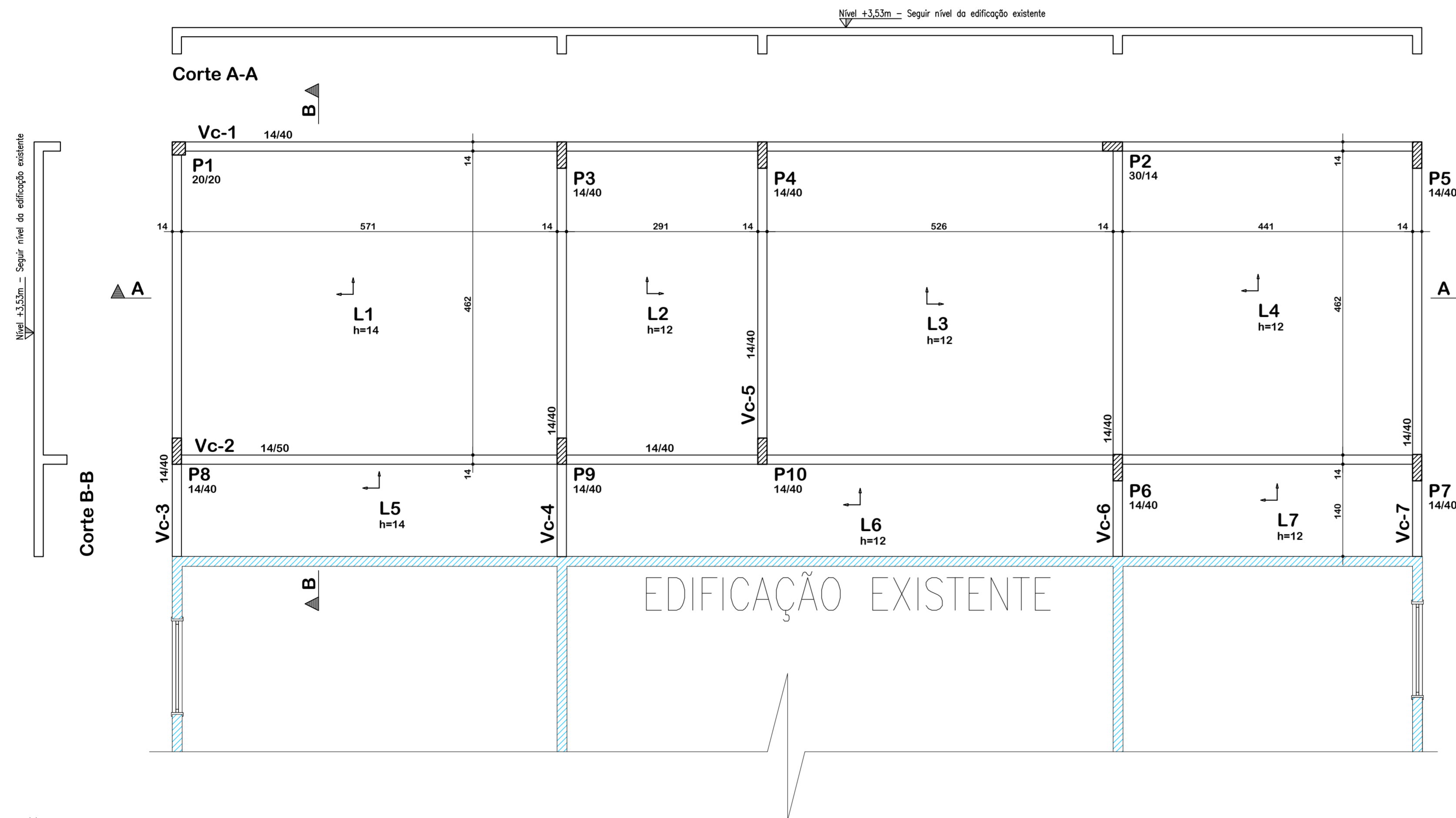
Planta de formas: Cobertura Escala: 1:50
