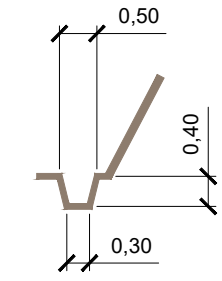
DETALHE CANALETA DE TOPO ESCALA: 1/100 DECLIVIDADE MÍNIMA DA CANALETA: 2%
