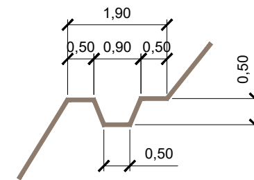
DETALHE CANALETA DE TOPO
