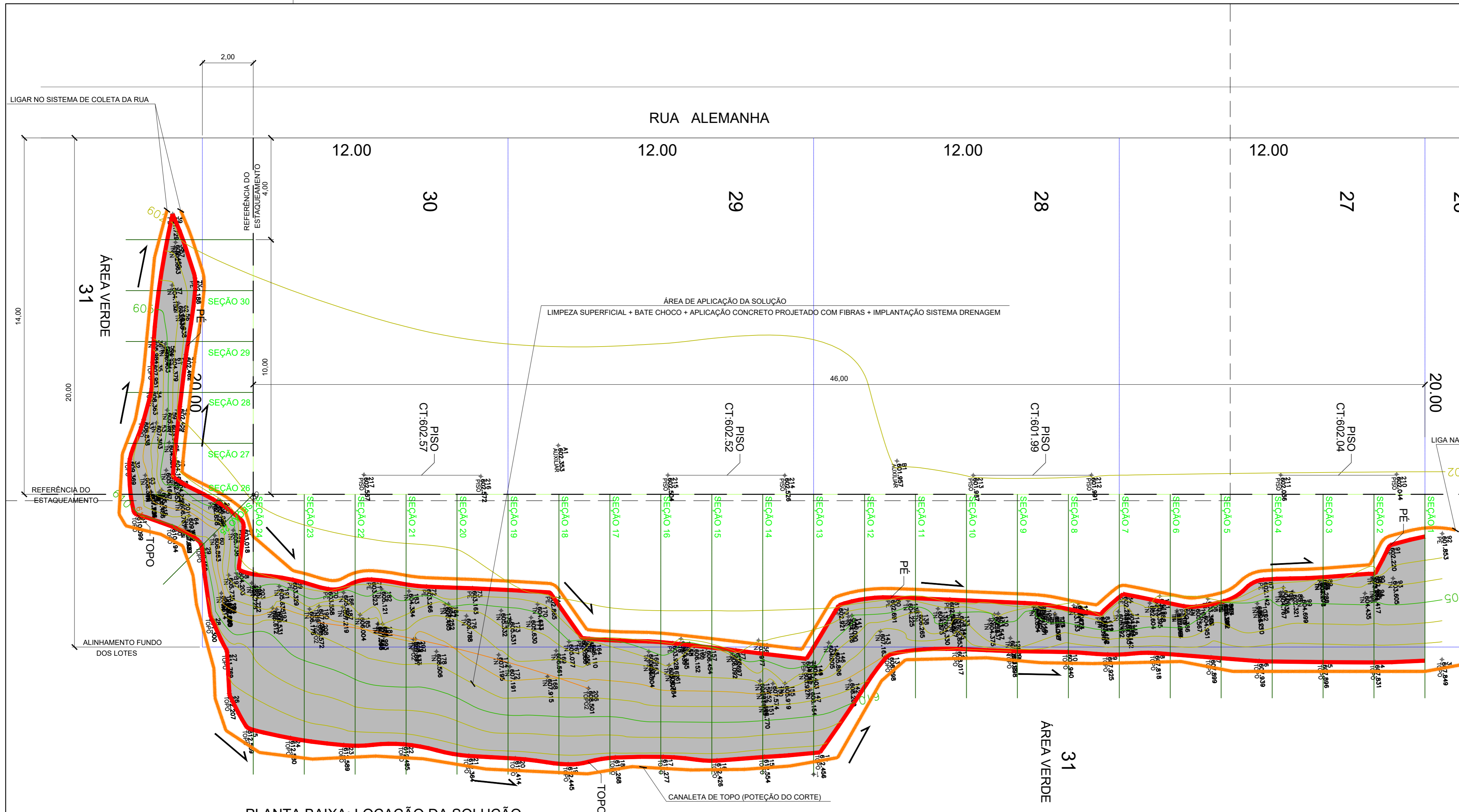
PLANTA BAIXA: LOCAÇÃO DA SOLUÇÃO ESCALA: 1/100
