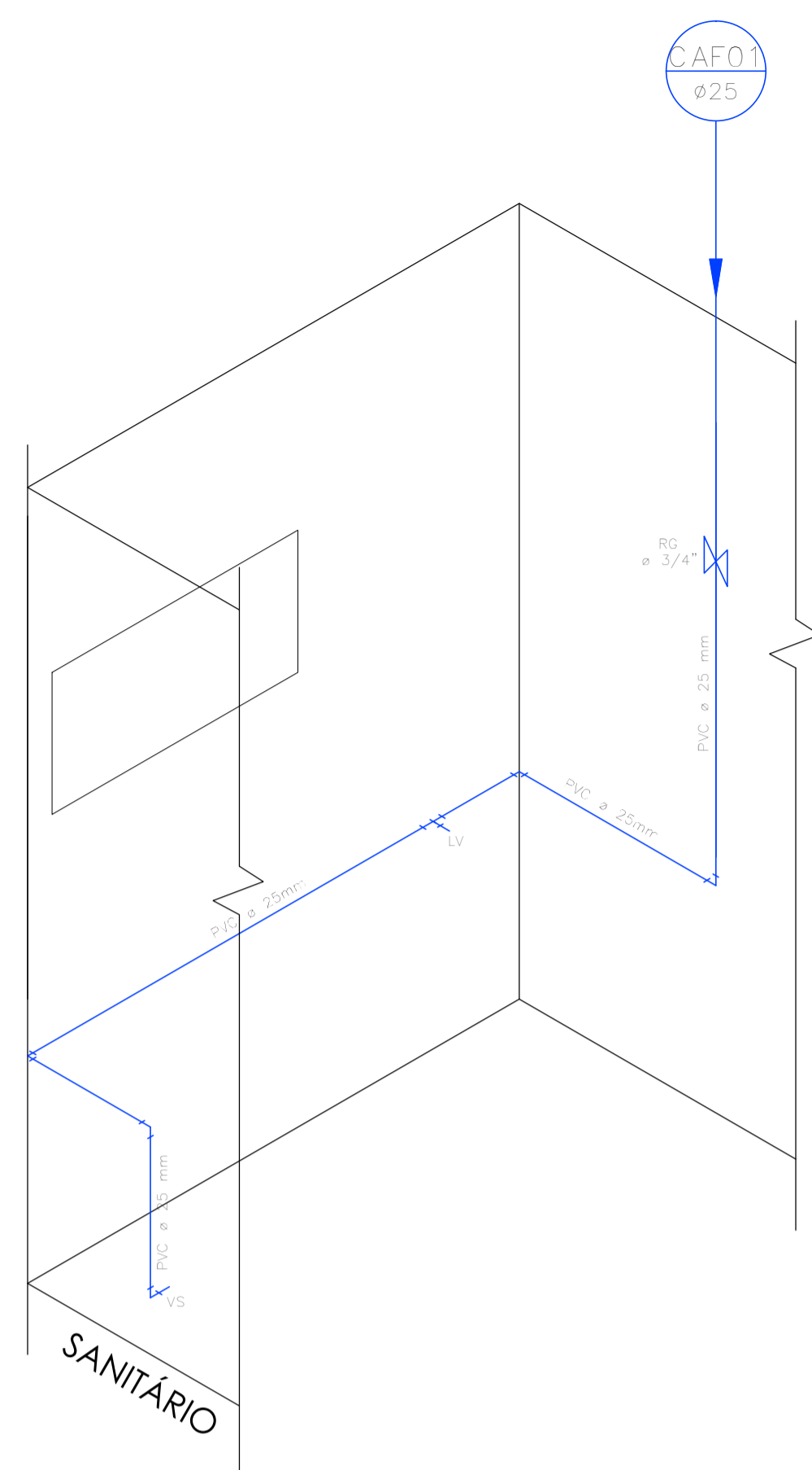
DETALHES ISOMÉTRICOS ESCALA 1:25
