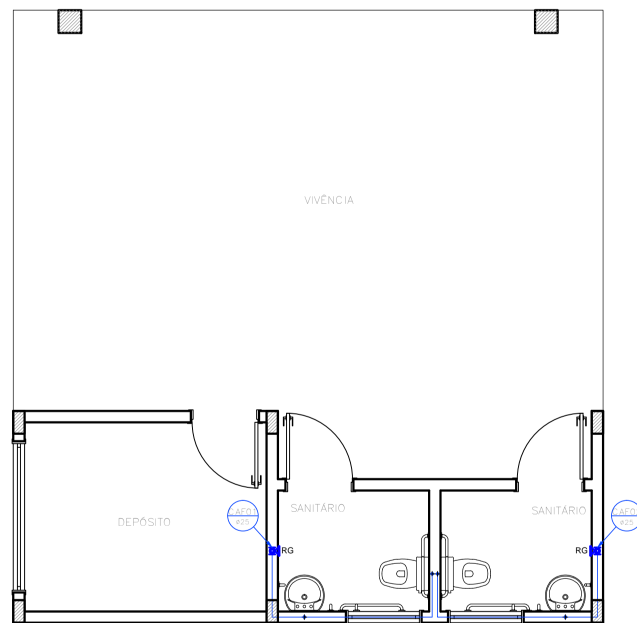
PLANTA BAIXA - HIDRÁULICO ESCALA 1:50
