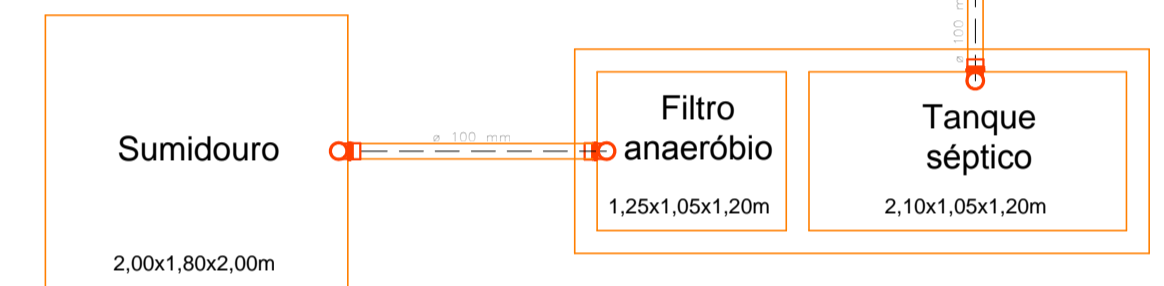
PLANTA BAIXA - SANITÁRIO ESCALA 1:50
