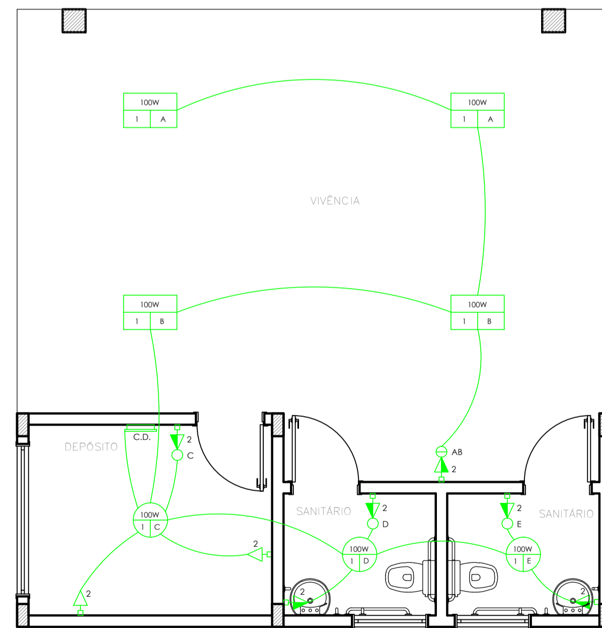
PLANTA BAIXA - ELÉTRICO ESCALA 1:50
