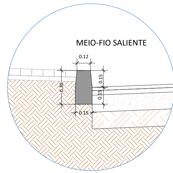
DETALHE 01 ESC.: 1:20
