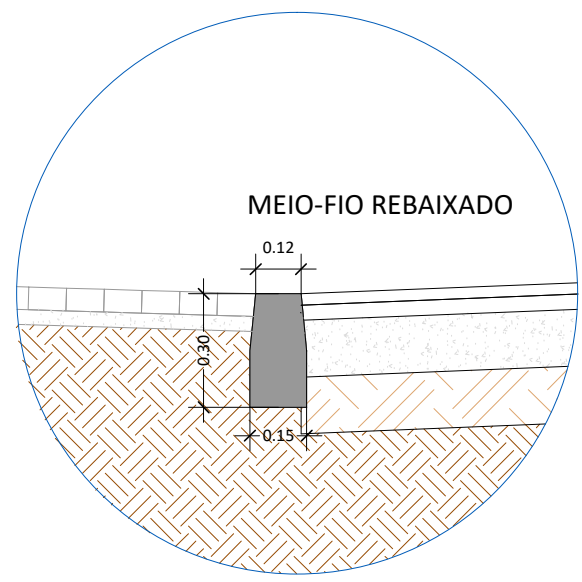
DETALHE 02 ESC.: 1:20
