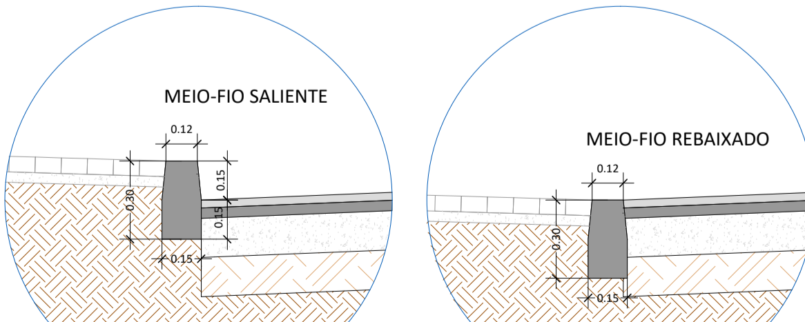
DETALHE 01 ESC: 1:20 DETALHE 02 ESC: 1:20
