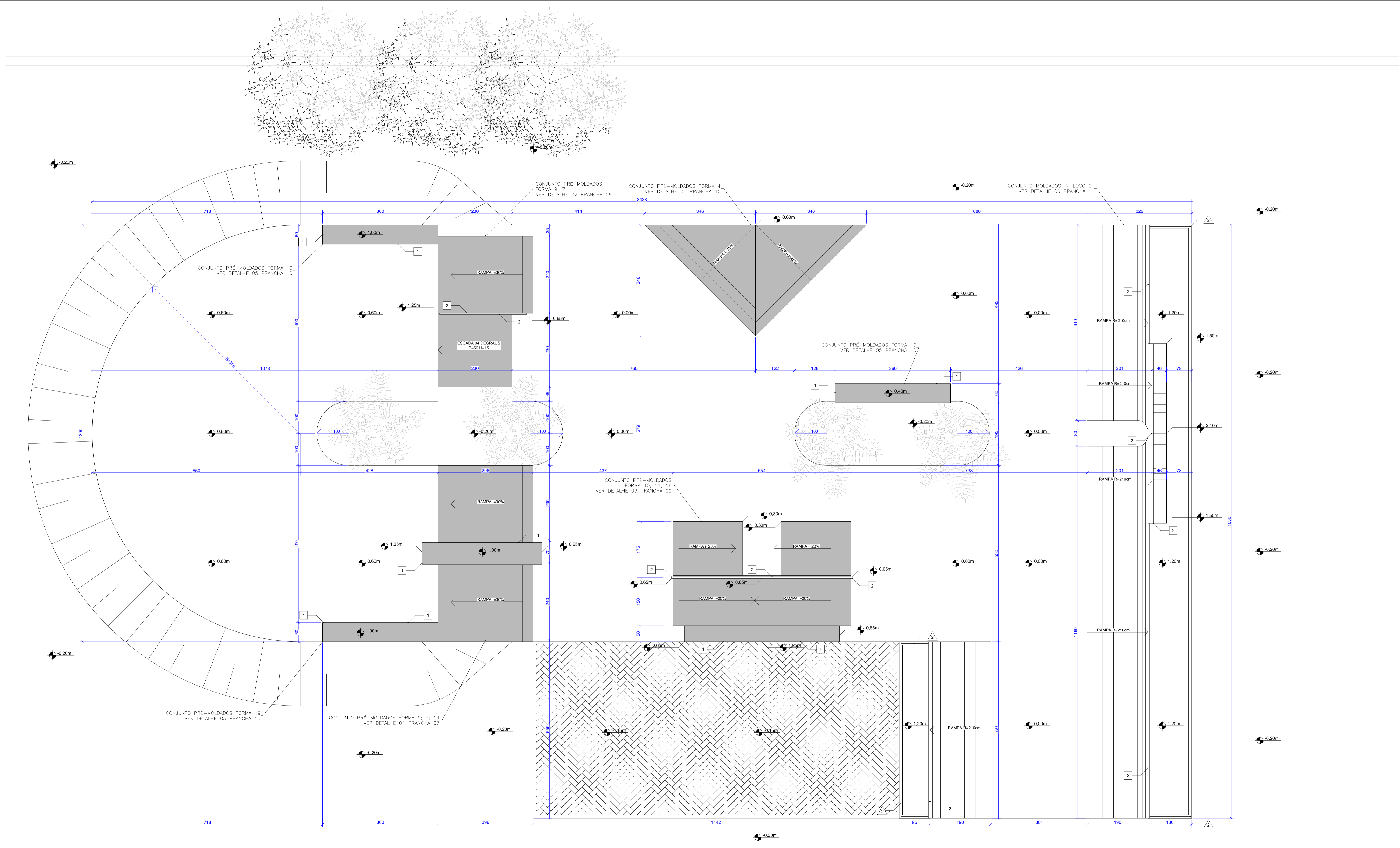
02 PLANTA BAIXA esc: 1:50
