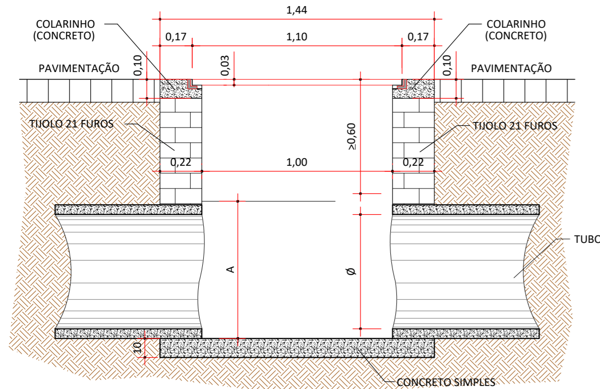
CORTE LONGITUDINAL (A A) ESC.: 1:20
