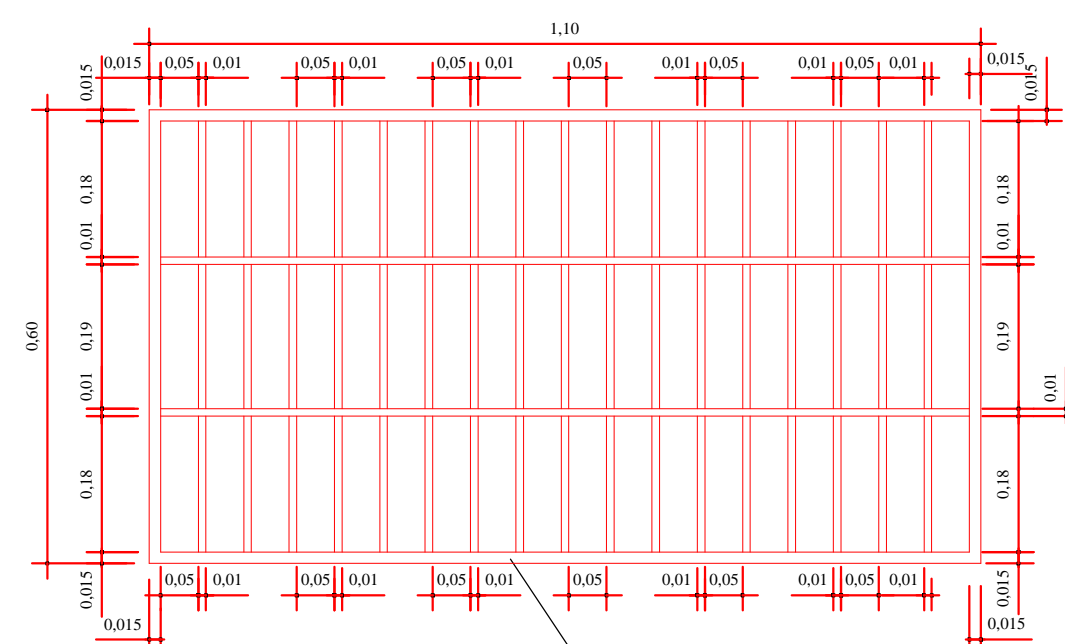
PLANTA - GRELHA ESC.: 1:10
