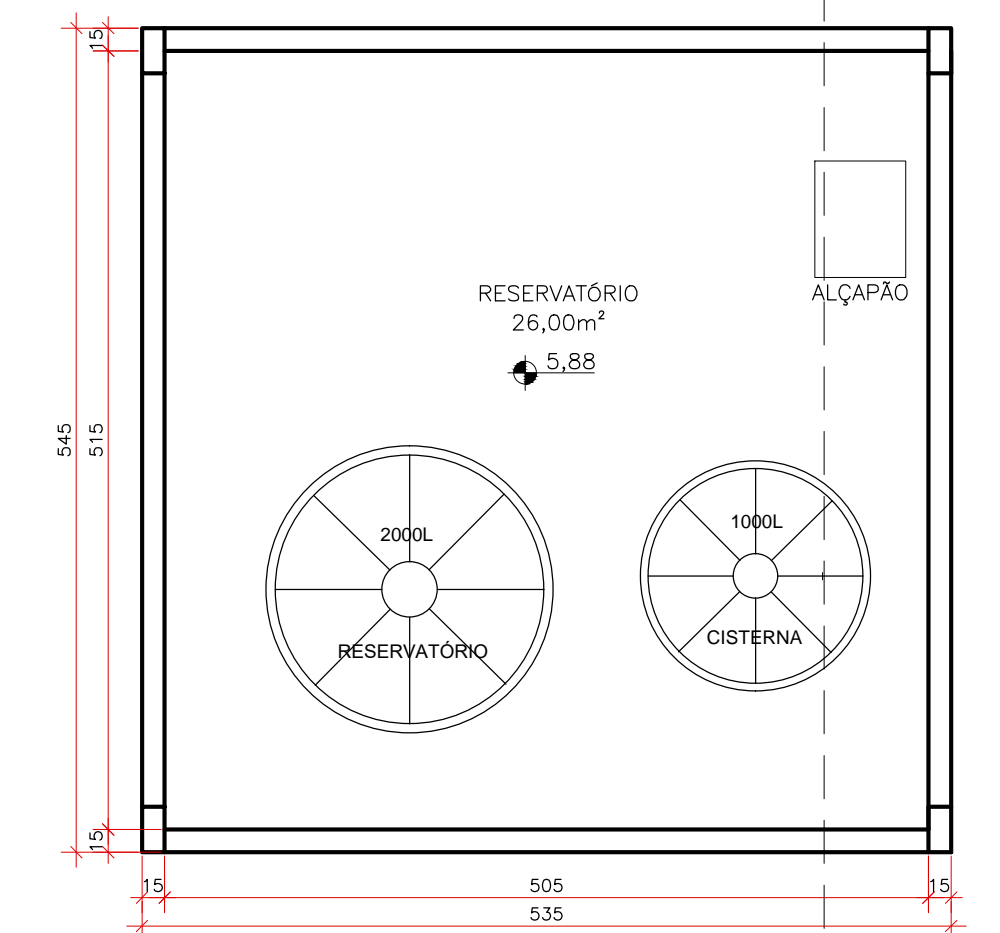
PLANTA BAIXA RESERVATÓRIO ESC.: 1:50
