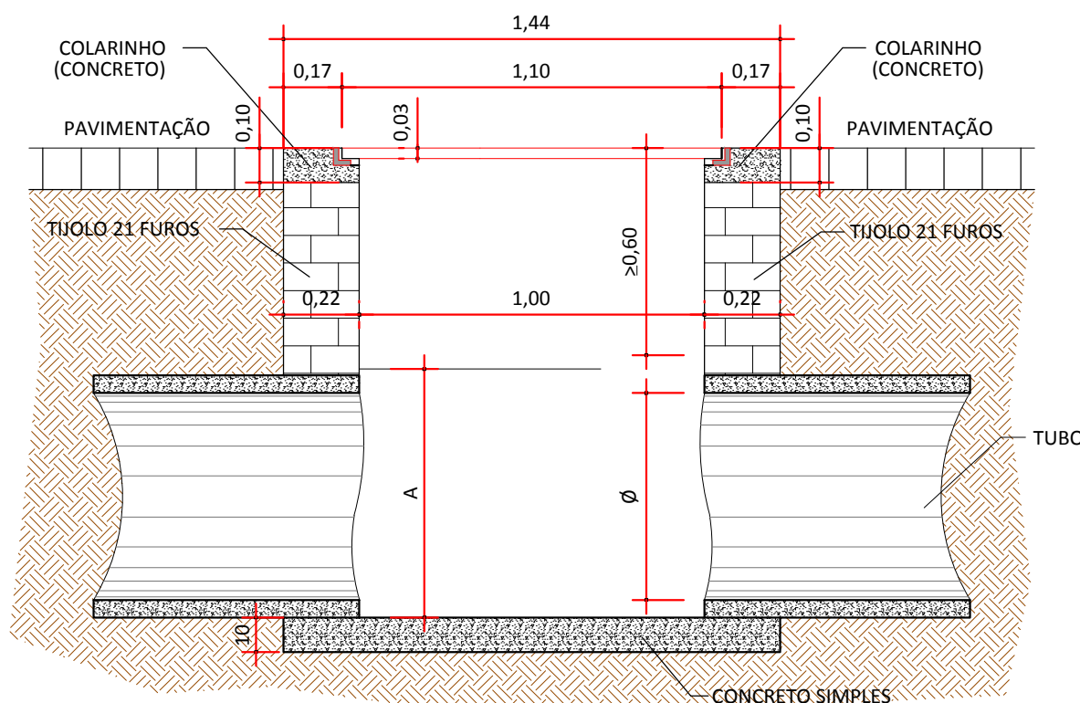
CORTE LONGITUDINAL (A A) ESC.: 1:20
