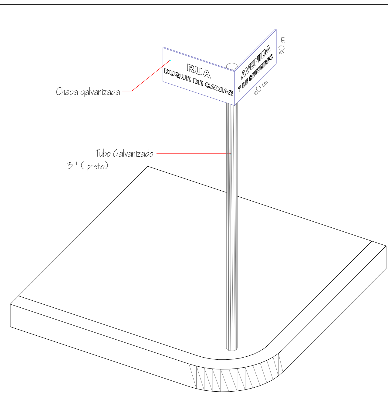
VISTA - PLACA COM NOMES DE RUAS ESC: 1/25
