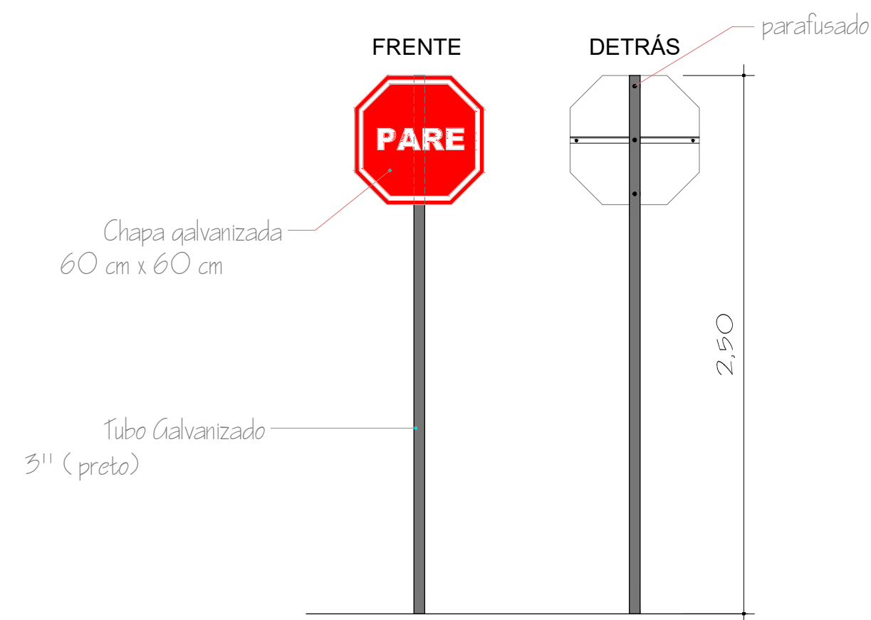
VISTA - PLACA SINALIZAÇÃO ESC: 1/25
