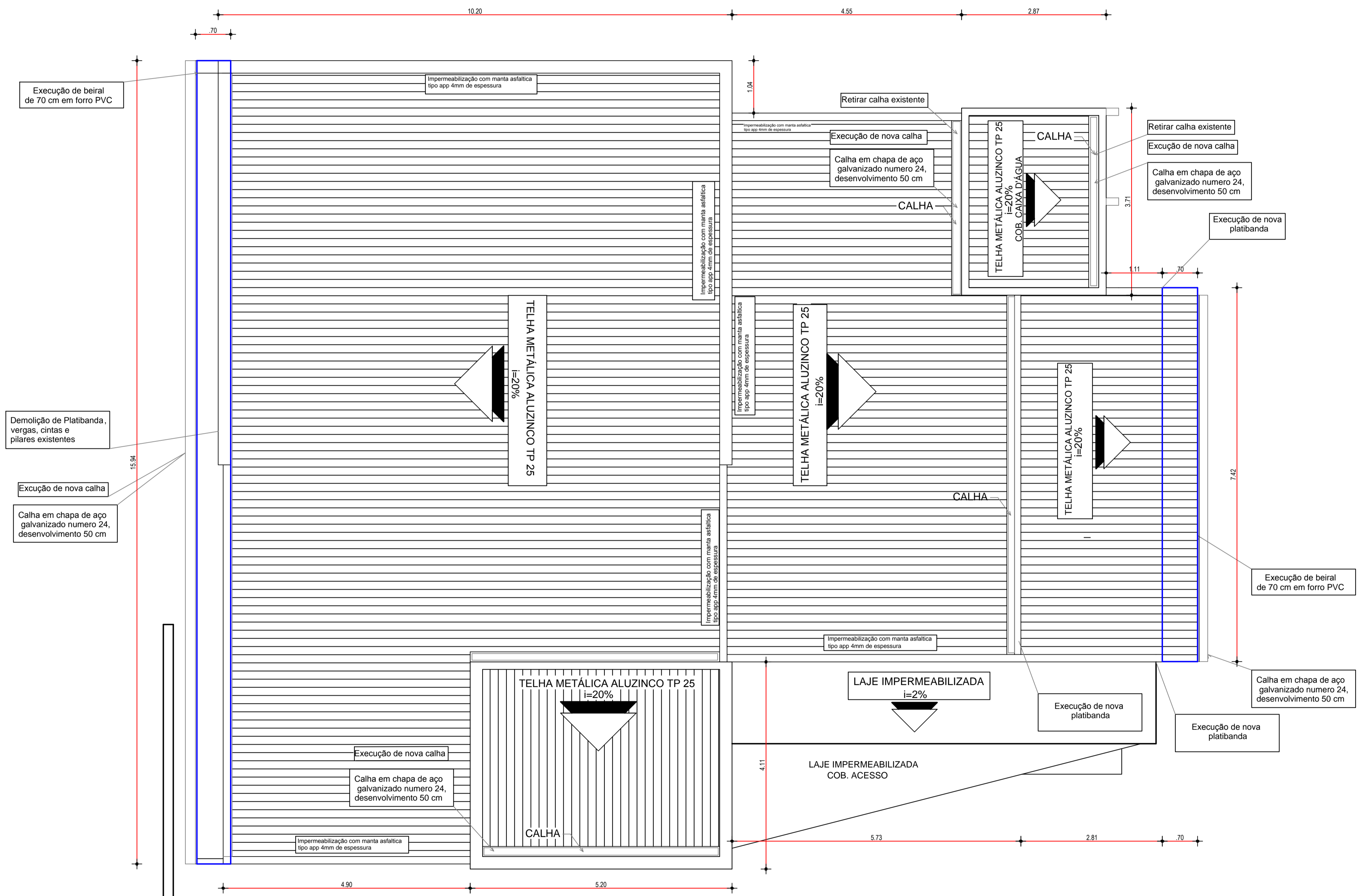
PLANTA DE COBERTURA ESCALA = 1:50
