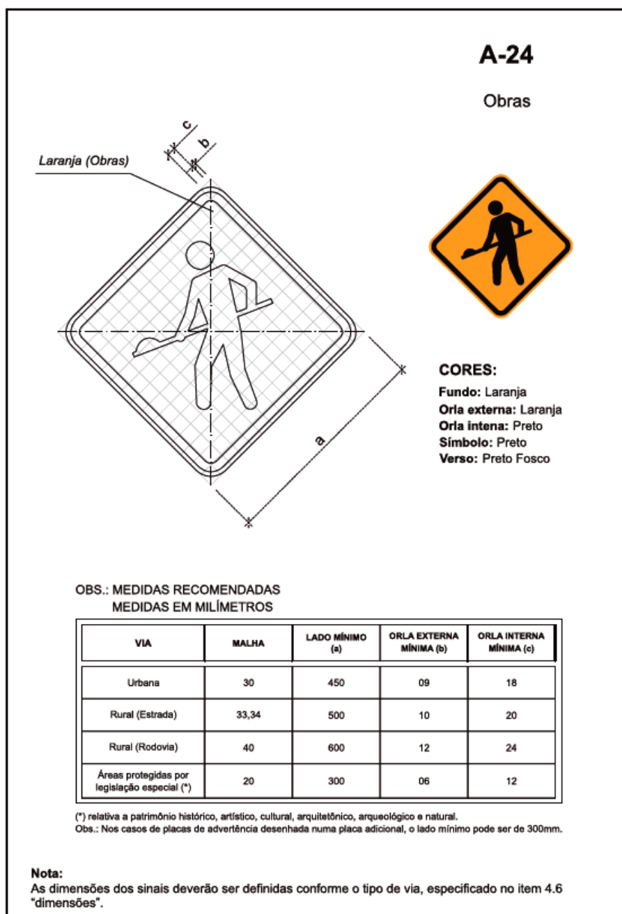
Figura 3: Placa de sinalização de obra; Fonte: Manual Brasileiro de Sinalização de trânsito - CONTRAN
