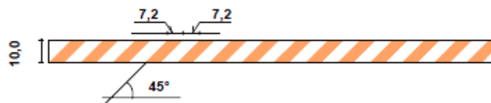
Figura 2: Fita zebraada; Fonte: Manual de Sinalização Urbana - CET;
