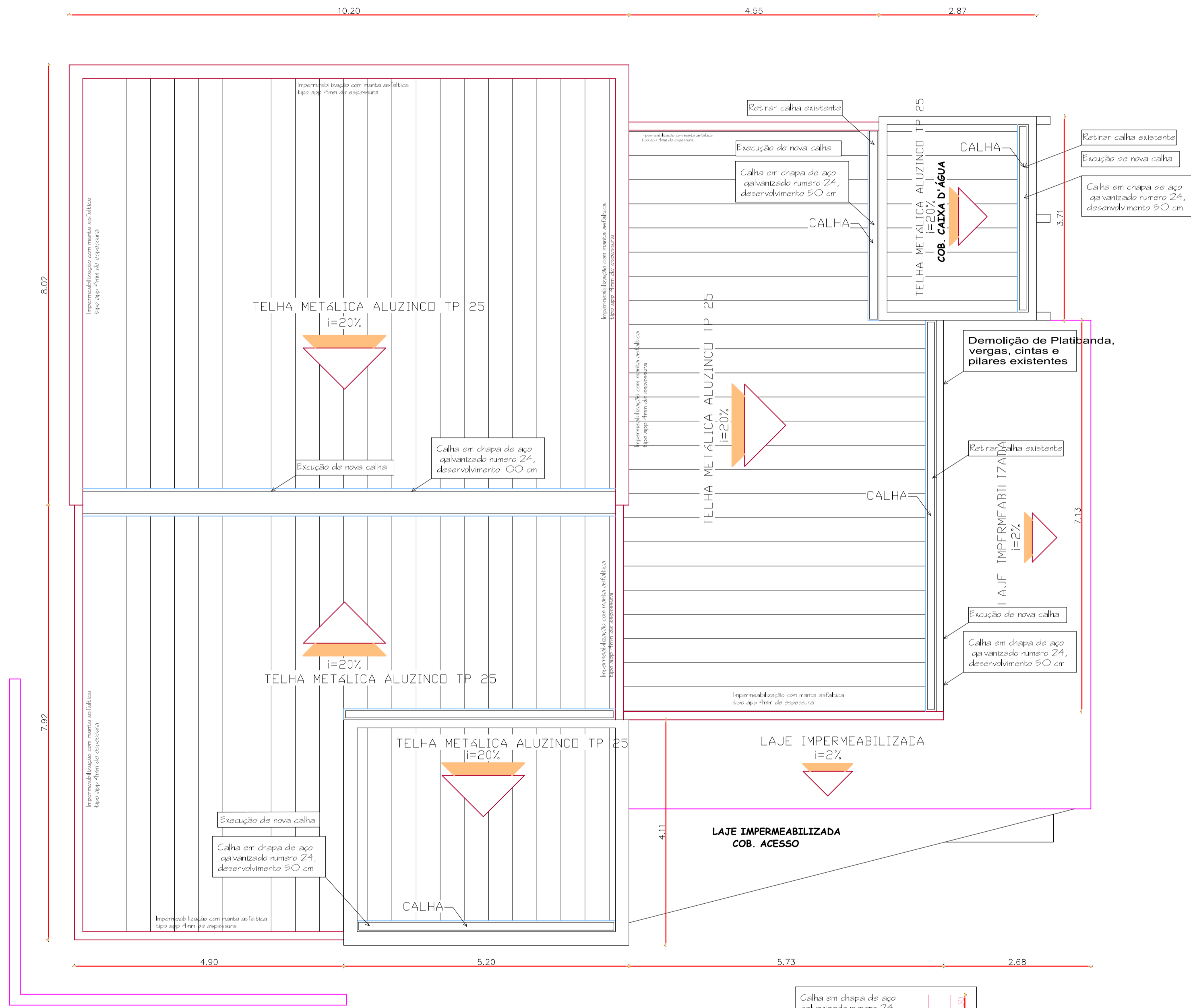
PLANTA DE COBERTURA ESCALA = 1:50
